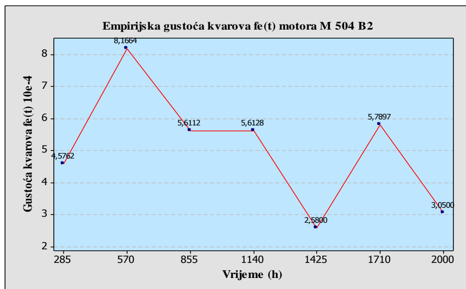
Slika 4.9 Empirijska funkcija gustoće kvara dizelskog motora M 504 B2
