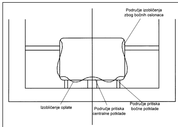
Slika 33. Moguće deformacije na oplati broda zbog reakcije potklada i podupirača
