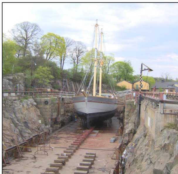
Slika 1. Suhi dok u Becholmenu u okolici Stockholma
