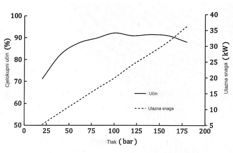
Dijagram 5.3 - Cjelokupni učin zupčaste pumpe pri brzini od 1500 o/min
