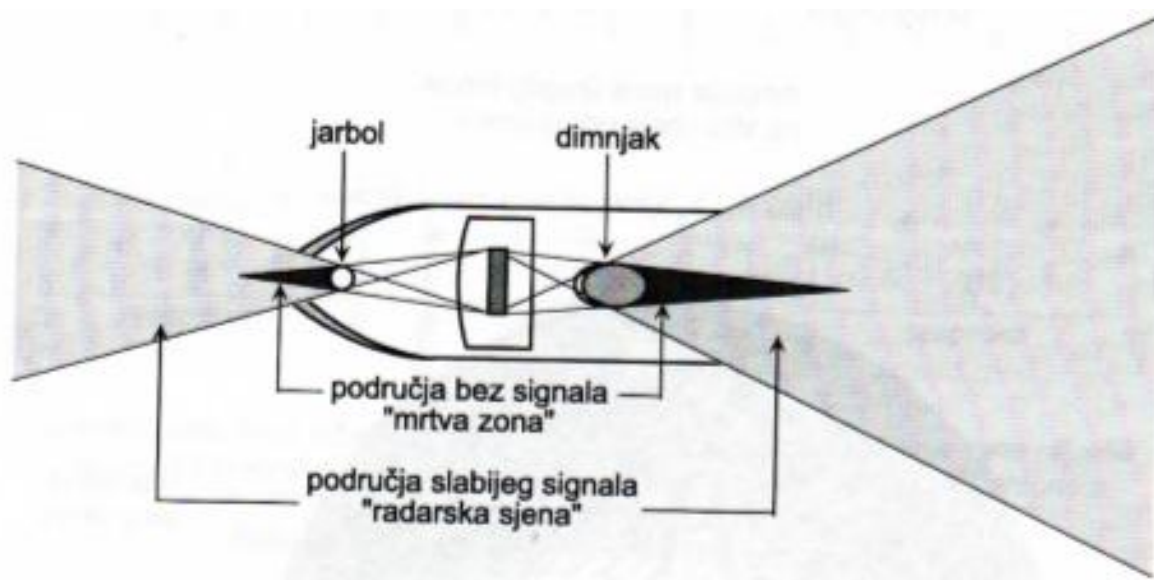
Slika 17. Radarske sjene i "slijepa" područja
