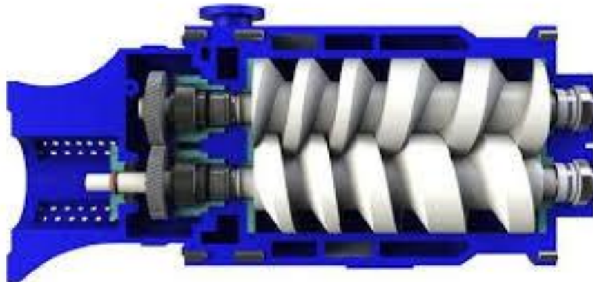
Slika 4: rotacijska pumpa (vijčana)
