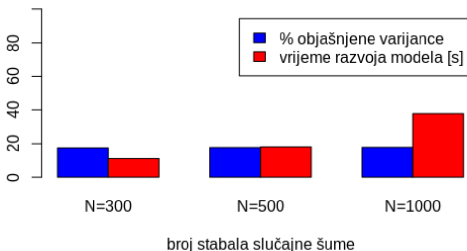
Slika 37. Usporedba računalne učinkovitosti razvoja modela slučajne šume
