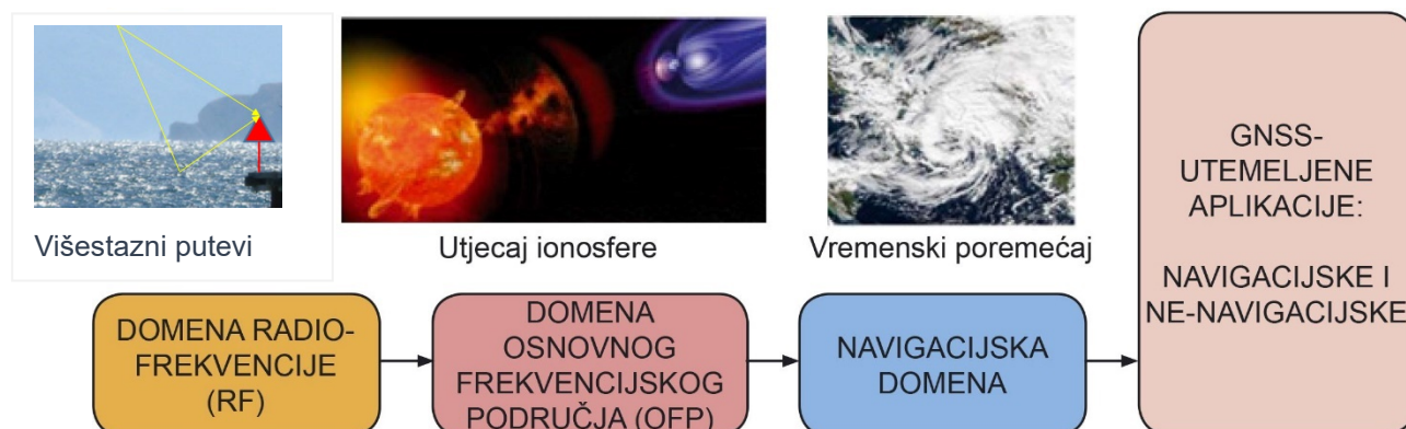
Slika 14. Izloženost satelitskog navigacijskog prijamnika raznim utjecajima okoline
