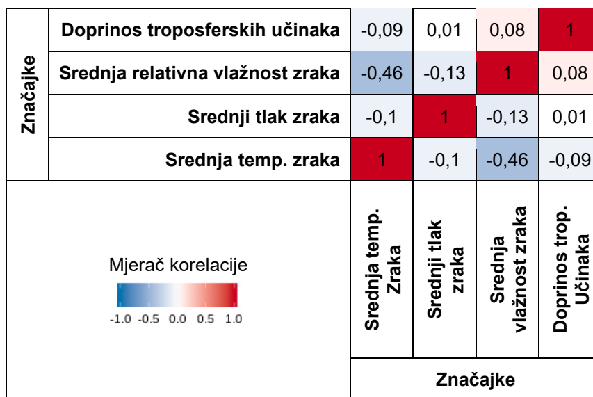
Slika 31. Korelacijski dijagram ciljne varijable i prediktora, izvedeno vlastitom programskom podrškom u okruženju za statističko računarstvo R i uz korištenje R knjižnice DataExplorer
