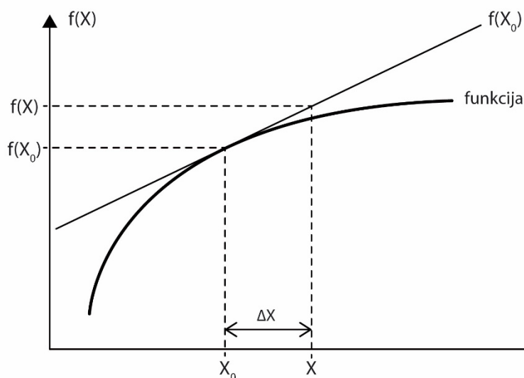
Slika 13. Linearizacija nelinearne funkcije u okolišu točke (x_0, f(x_0)) primjenom Taylorovog reda (prema: Higham, N J i suradnici, 2015)
