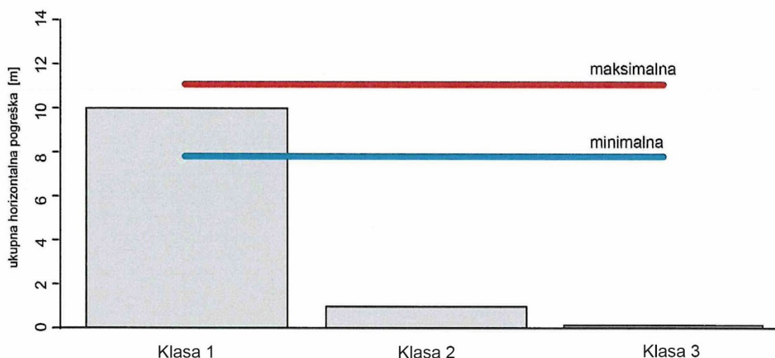
Slika 40. Preslikavanje graničnih vrijednosti ukupne pogreške satelitskog određivanja položaja u pomorskoj površinskoj navigaciji, procijenjene pomoću stvarnog doprinosa uslijed troposferskih učinaka i uobičajenih vrijednosti ostalih doprinosa, na zahtjeve za točnost određivanja položaja klase primjena u pomorskoj površinskoj navigaciji
