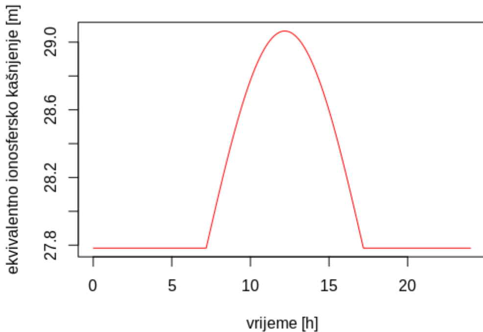
Slika 21. Klobucharov model dnevnog hoda ionosferskog kašnjenja satelitskog signala za određivanje položaja
