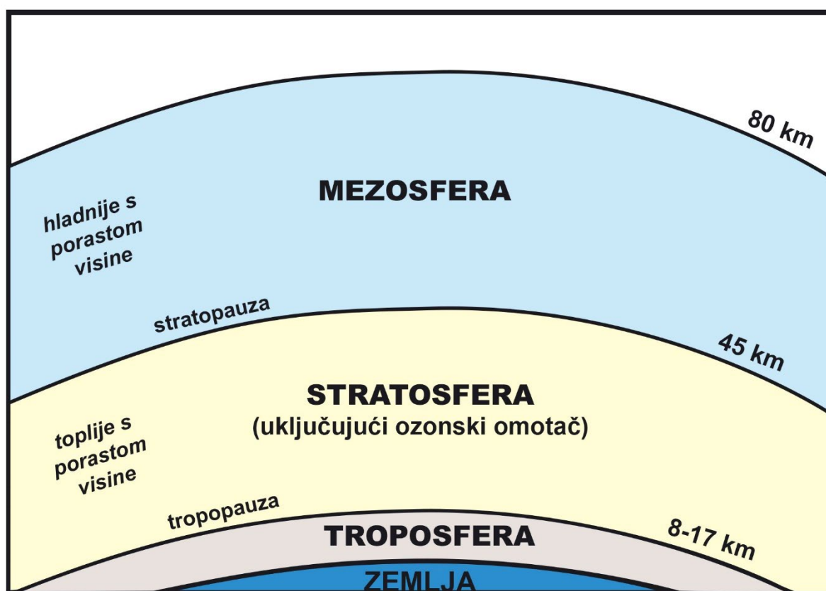
Slika 15. Vertikalni profil atmosfere (prema: Gelo, 2000)
