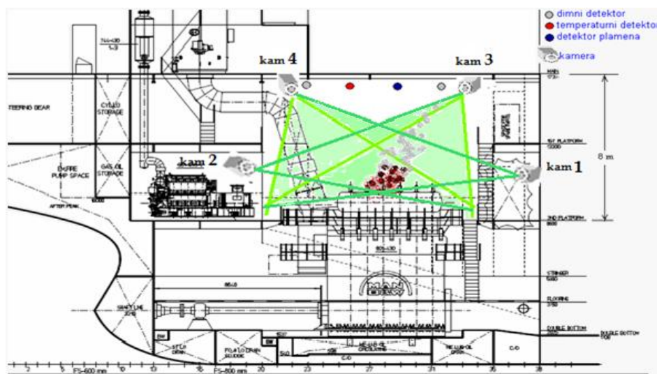
Slika 69: Pozicije IP kamere za test videodetekcije dima
