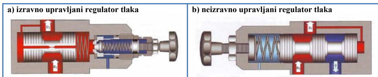
Slika 4-18. Ventili za reguliranje tlaka [6, p. 100]
