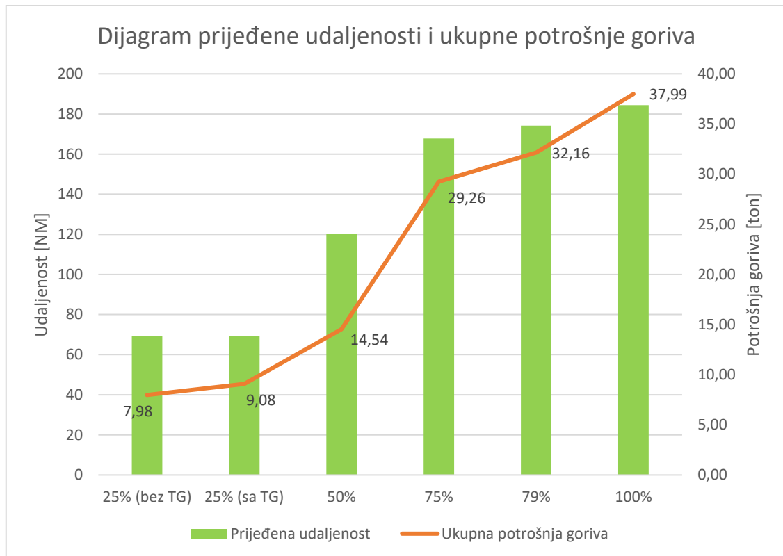
Slika 9 - Prikaz prijeđene udaljenosti i ukupne potrošnje goriva
