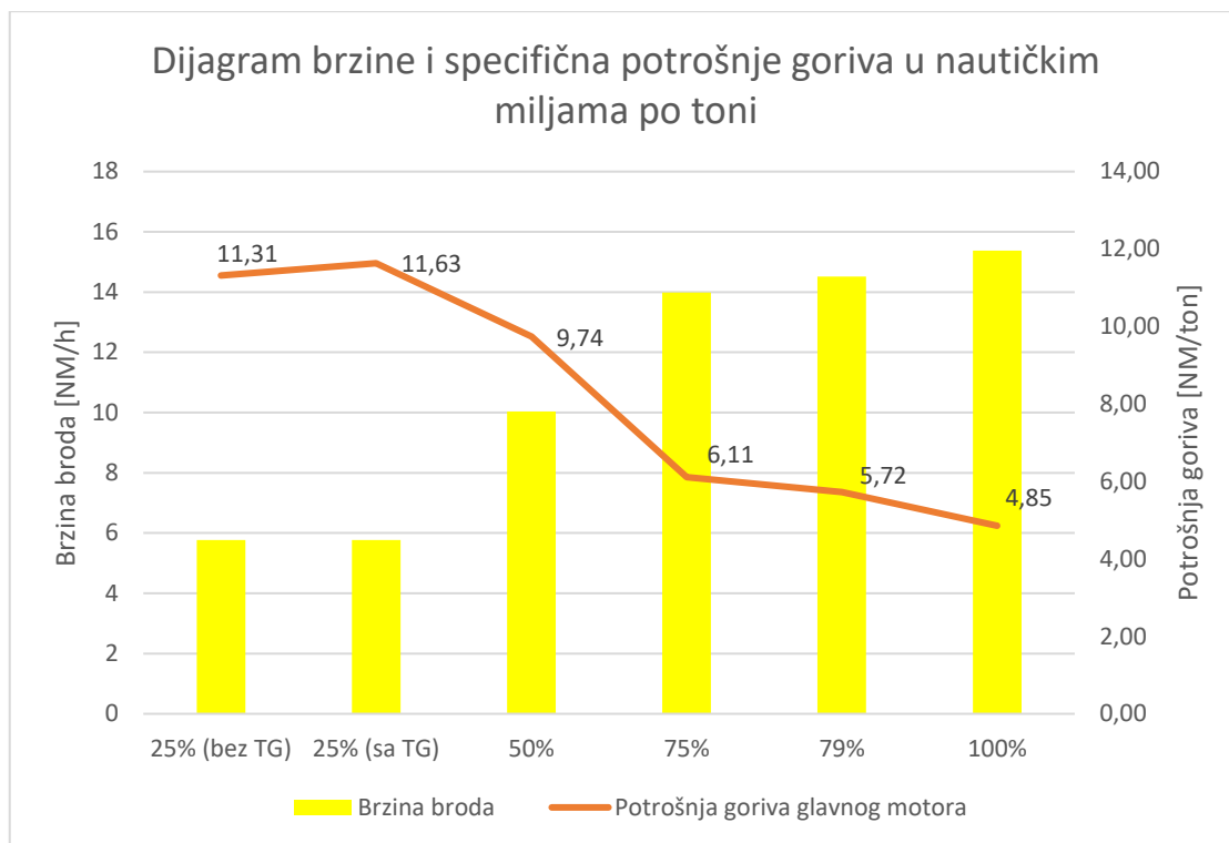
Slika 10 - Prikaz brzine i specifične potrošnje goriva
