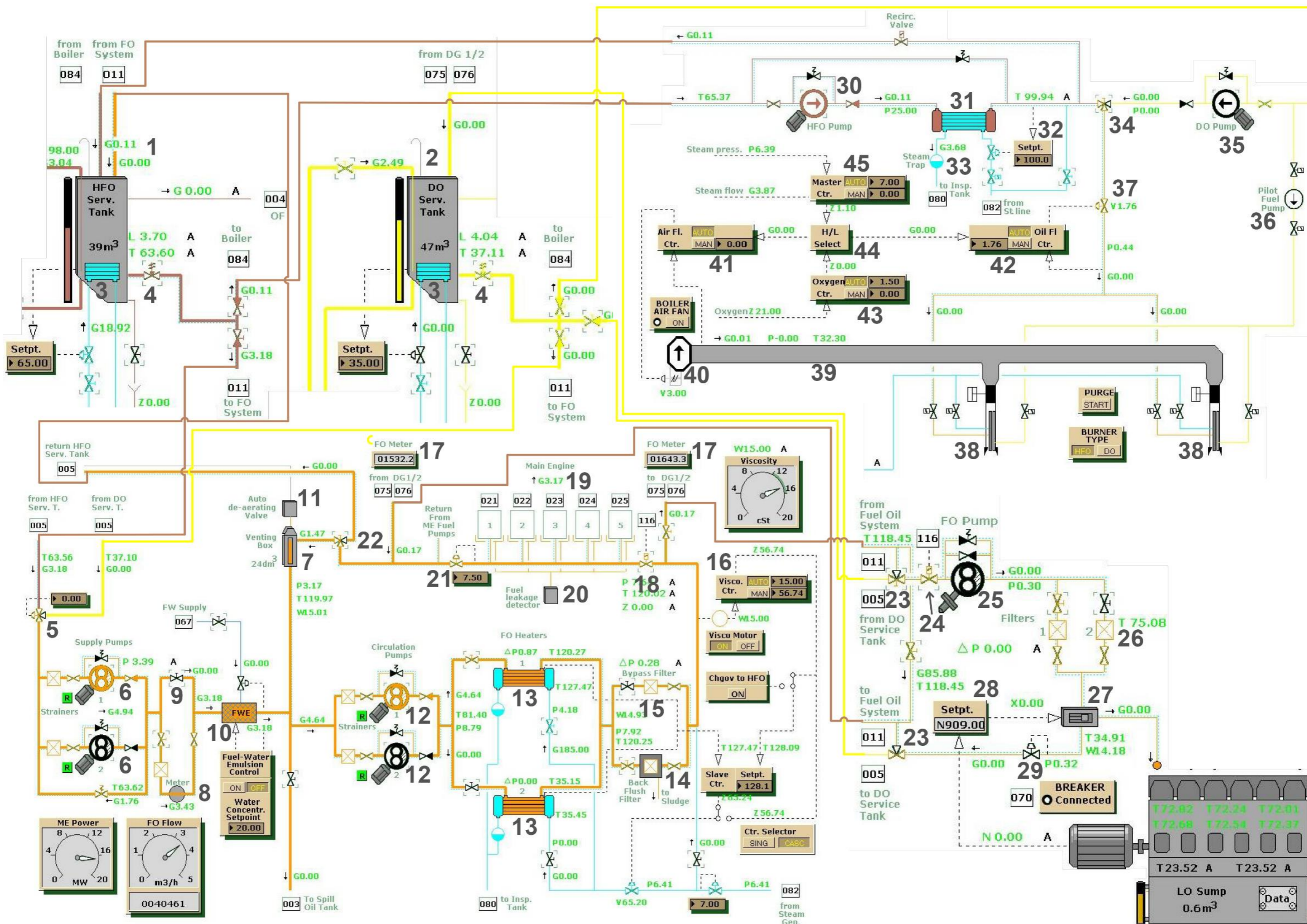
Slika 1 - Prikaz sheme goriva glavnog i pomoćnih motora te loženog generatora pare
