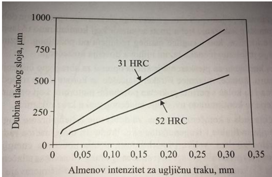
Slika 6. Ovisnost dubine tlačnog sloja o Almenovom intenzitetu za ugljičnu traku za čelike različitih tvrdoća
