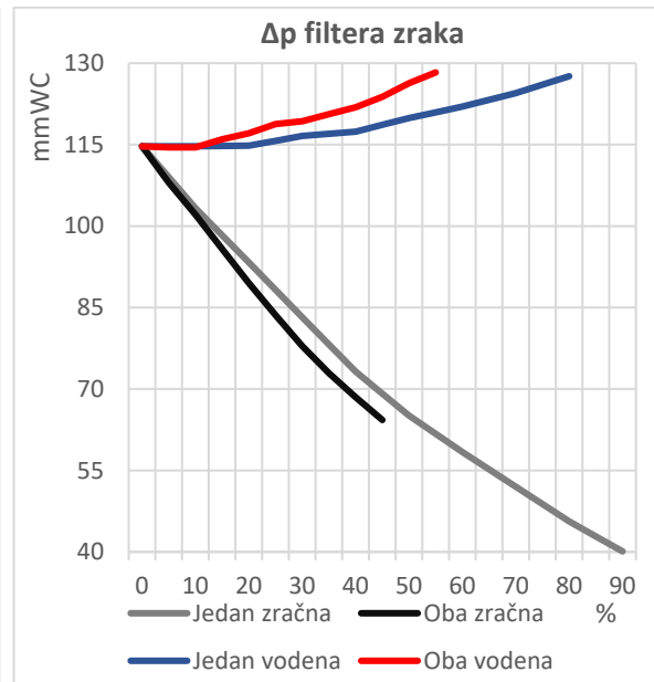
Slika 12. Δp filtra zraka
