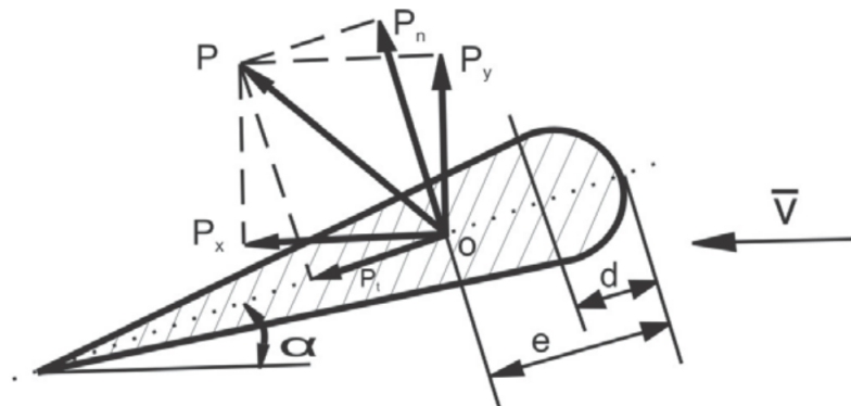
Slika 31. Prikaz sila pasivnog kormila
