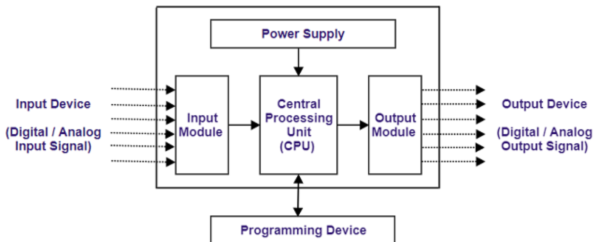
Slika 19: Blok dijagram PLC-a
