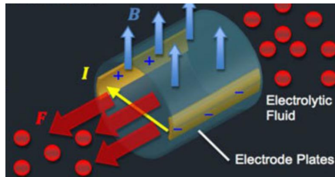
Slika 34. Pr1incip rada MHD propulzije
