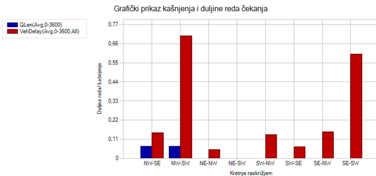
Grafikon 6. Prikaz kašnjenja i duljine reda čekanja na raskrižju R39 (na temelju stvarno izmjenenog signalnog plana)
