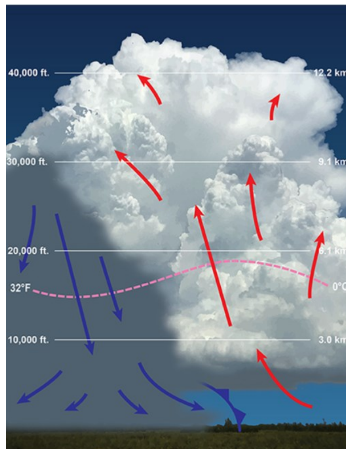
Slika 8. Zrela faza olujnog oblaka
