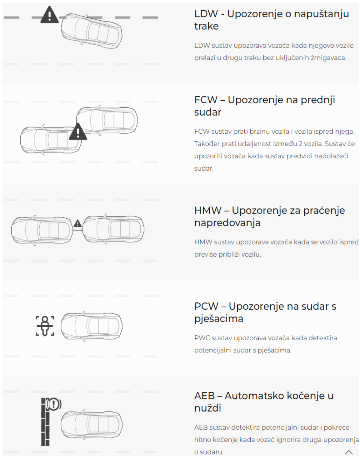
Slika 9. Funkcije ADAS-a
