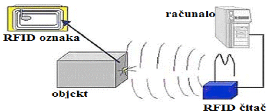
Slika 4. RFID sustav
