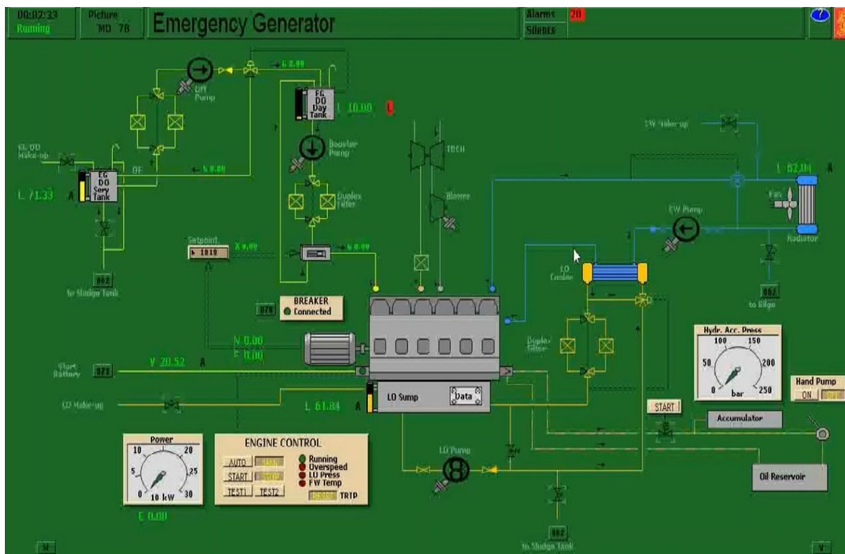
Slika 12. Shematski prikaz generatora za nužnost u Kongsberg simulatoru
