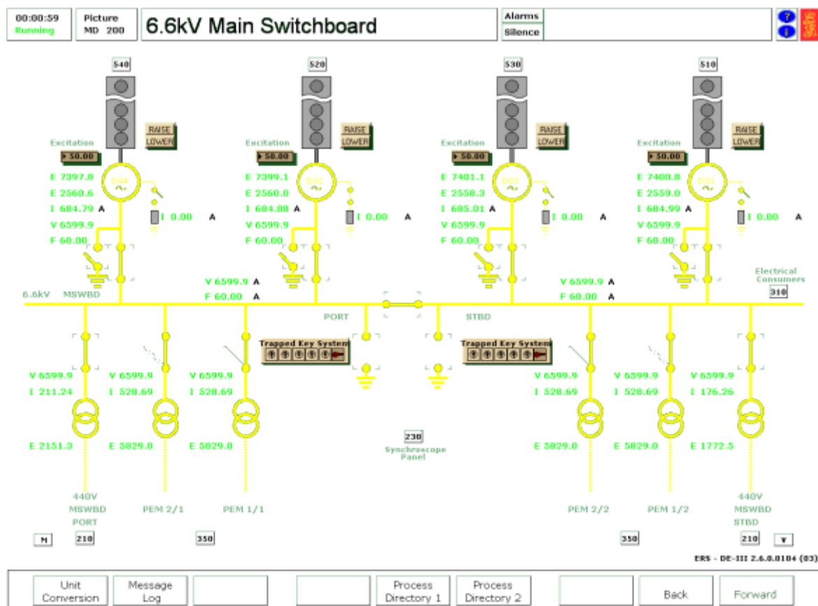
Slika 16. Jednopolna shema VN-GRP 6,6kV
