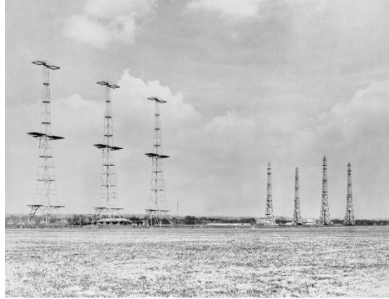
Slika 2.5 Britanski Chain Home sustav radarske detekcije.
