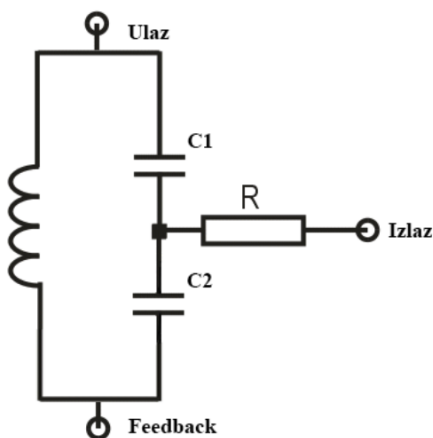
Slika 3.23 Colpitts oscilator
