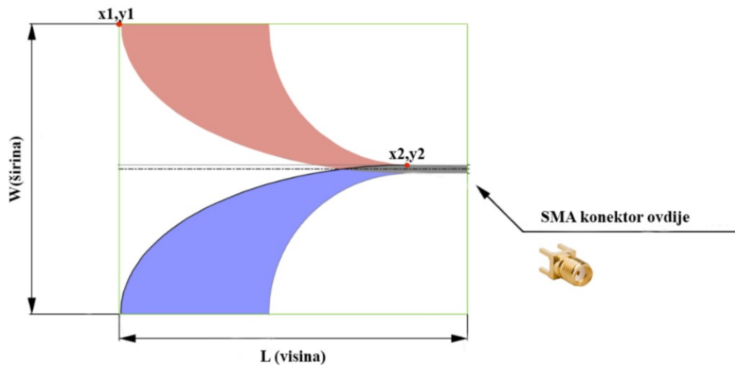
Slika 3.15 Antipodalna Vivaldi antena
