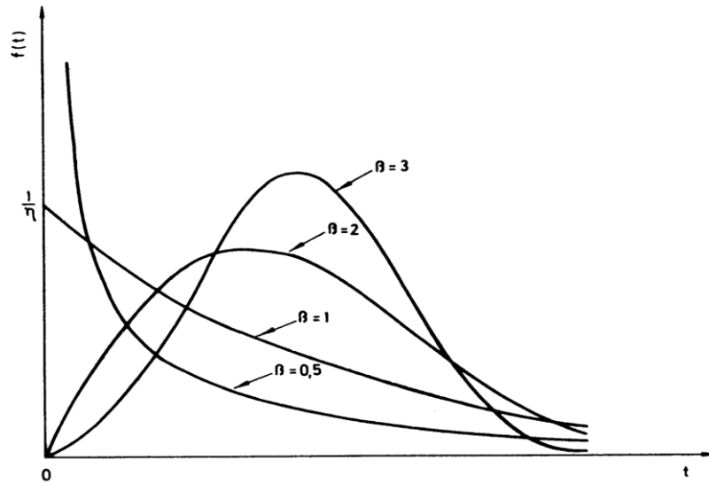
Slika 4.12 Funkcija gustoće kvarova f(t) za \gamma = 0, \eta = const. i razne vrijednosti parametra \beta
