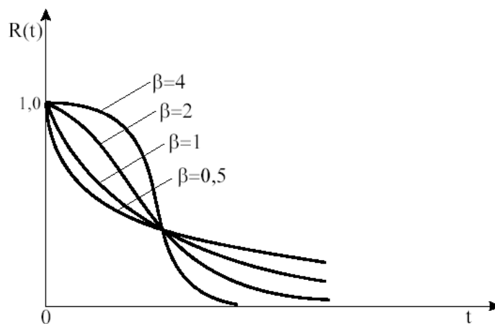
Slika 4.13 Funkcija pouzdanosti R(t) za \gamma = 0 i \eta = const. i razne vrijednosti parametra \beta
