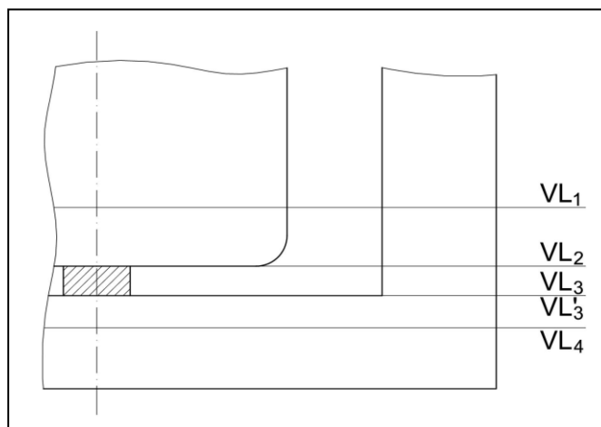
Slika 44. Karakteristične vodene linije pri dokovanju/izdokovanju broda
