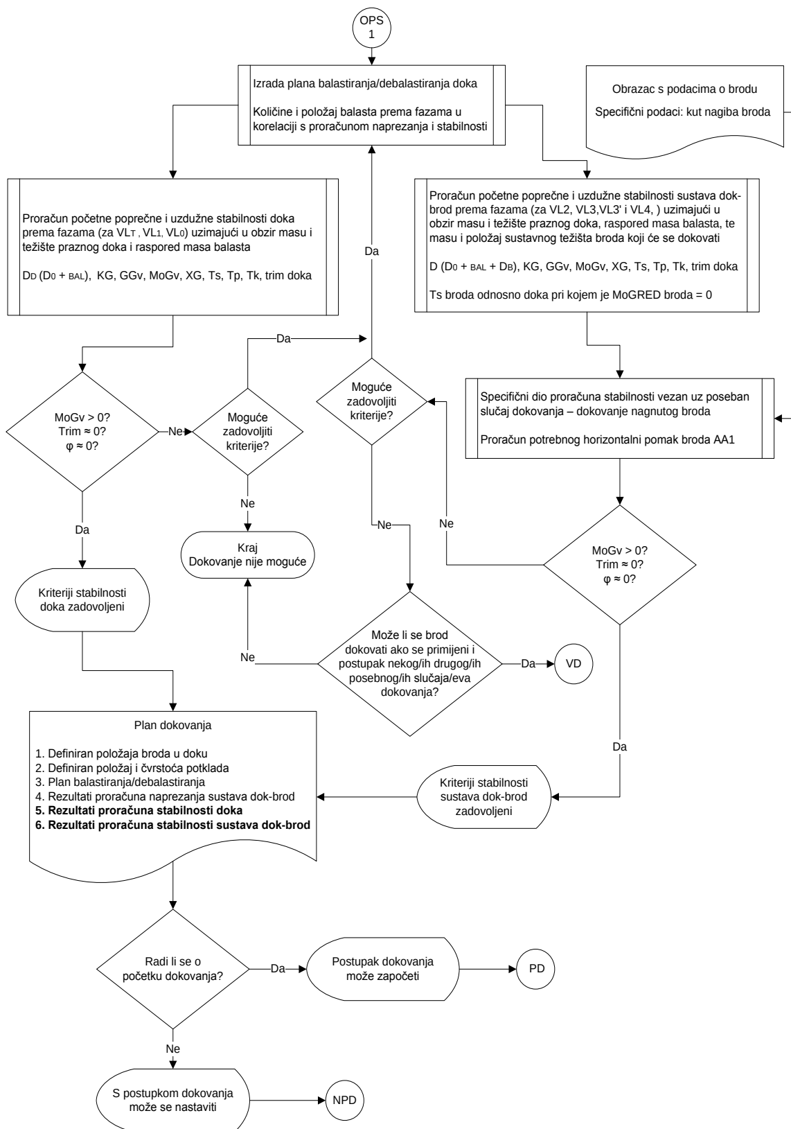
Slika 64. Dio konceptualnog modela određivanja parametara stabilnosti pri dokovanju nagnutog broda
