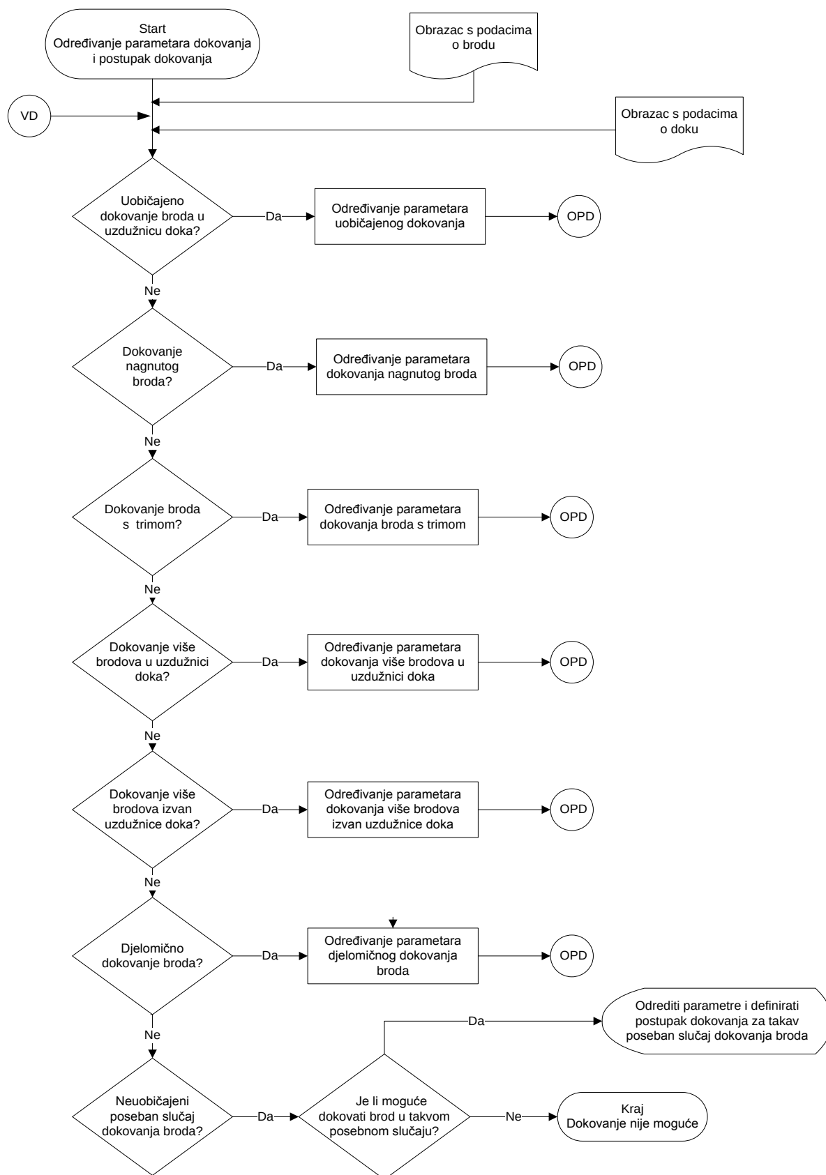
Slika 58. Konceptualni model definiranja vrste dokovanja
