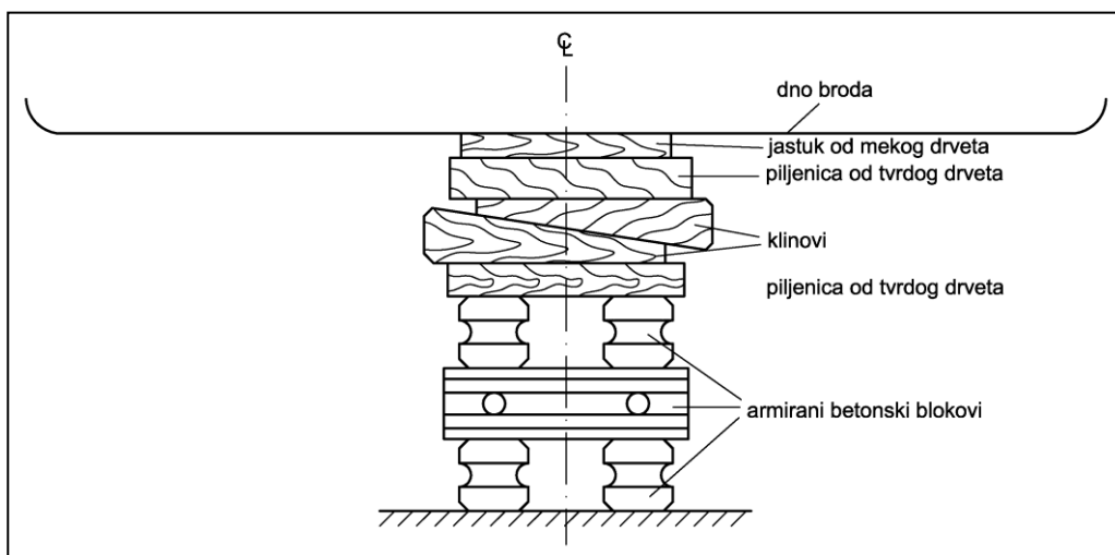
Slika 29. Kombinirana betonsko-drvena potklada
