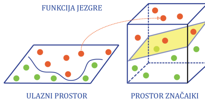
Slika 11. Transformacija pomoću jezgrene funkcije u strojevima potpornih vektora (SVM)
