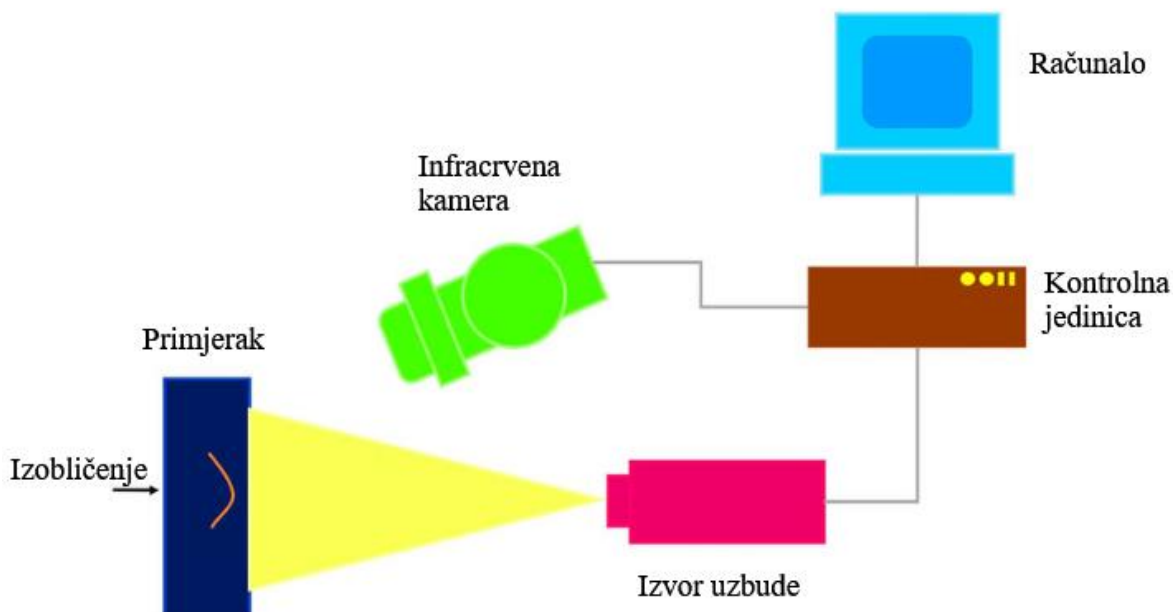
Slika 3: Aktivna termografija
