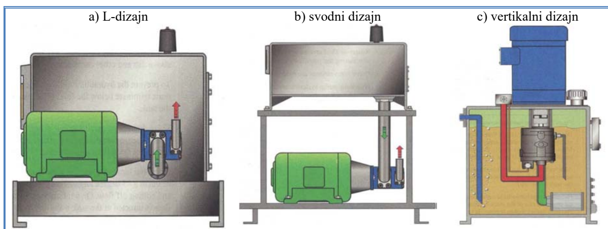
Slika 4-23. Dizajn spremnika ulja [3, pp. 96-98]
