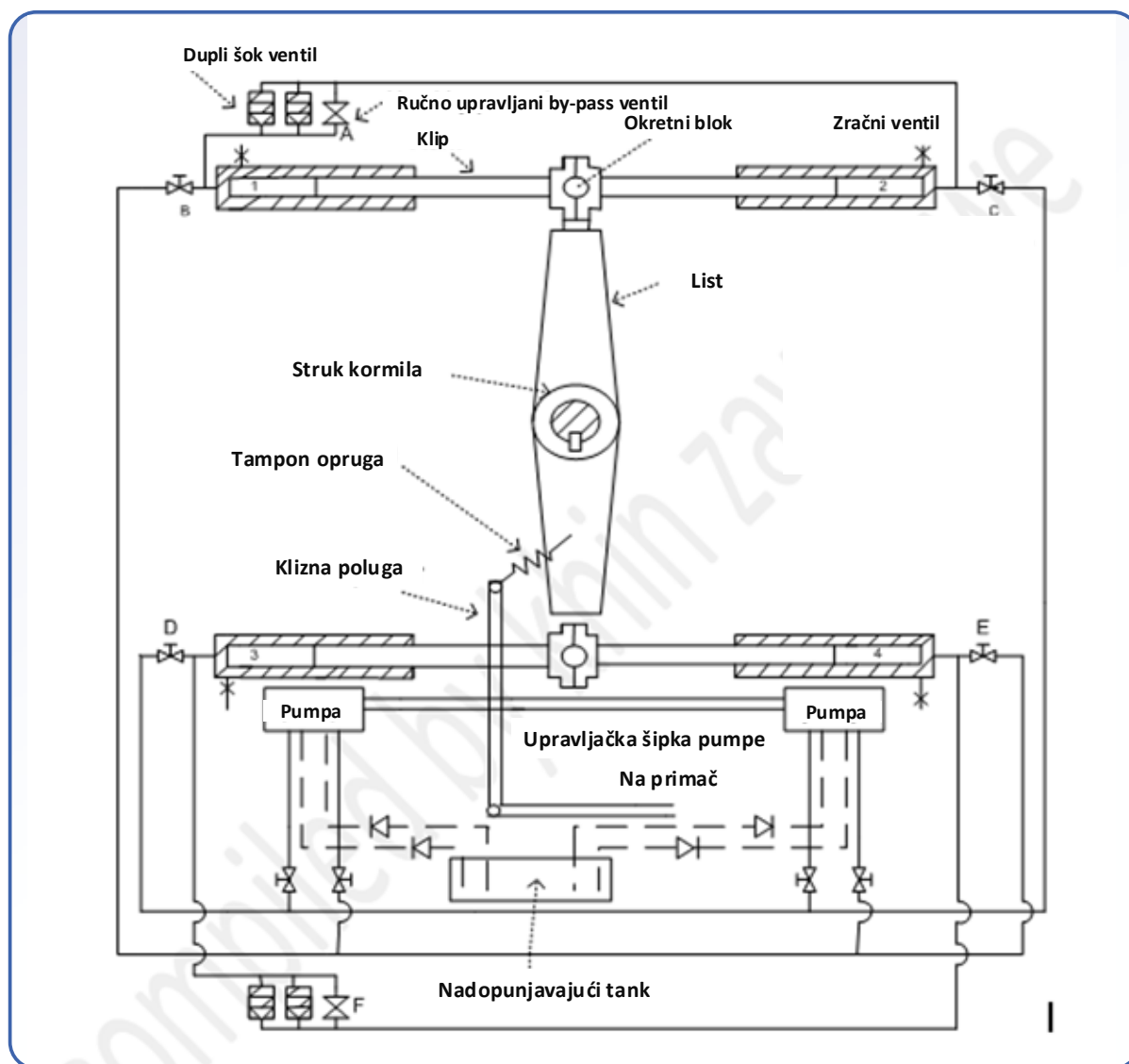
Slika 5-27. Sigurnosni elementi hidrauličkog klipnog kormilarskog uređaja
