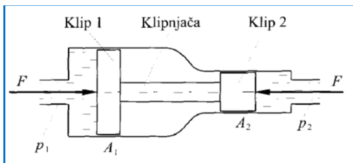
Slika 2-3. Princip pretvorbe tlaka
