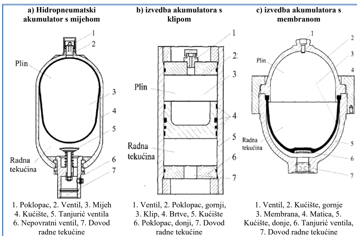
Slika 4-25. Hidropneumatski akumulatori s razdjelnim elementom [2, p. 201]
