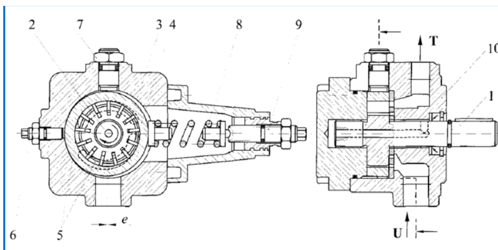
(1) pogonsko vrtilo, (2) rotor, (3) krilce, (4) odzivna staza statora, (5) radne komore, (6) vijak (7) vijak, (8) opruga, (9) vijak za regulaciju i (10) razvodna ploča.
