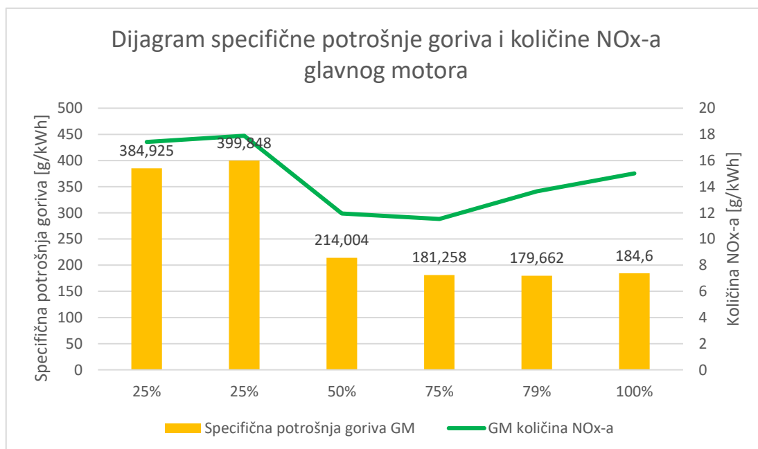
Slika 12 - Prikaz specifične potrošnje goriva i količine NO x -a glavnog motora
