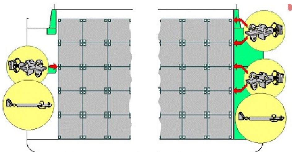
Slika 22 Učvršćivanje blokova kontejnera stabilizacijom
