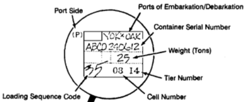
Slika 29 Identifikacijske oznake kontejnera
