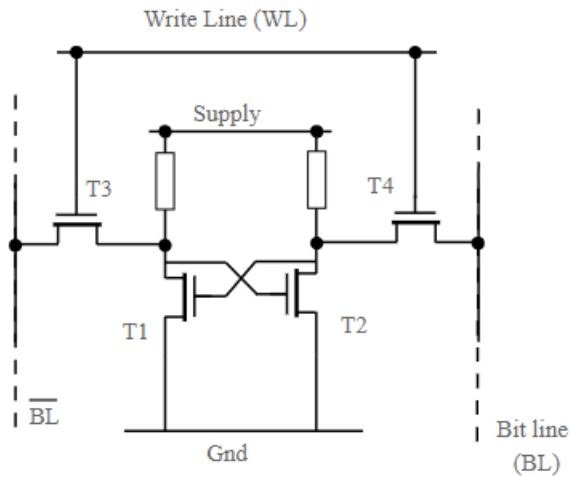
Slika 1. Struktura SRAM memorijske ćelije sa četiri tranzistora
