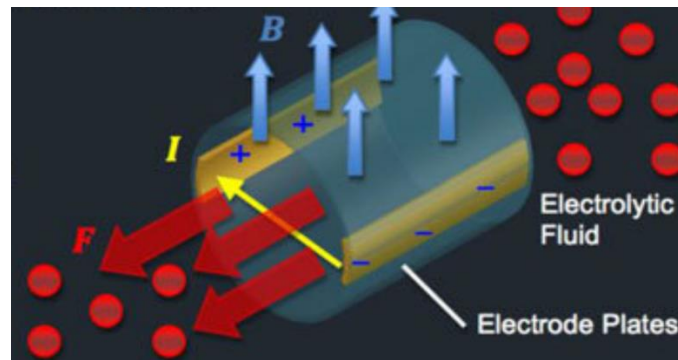
Slika 34. Princip rada MHD propulzije
