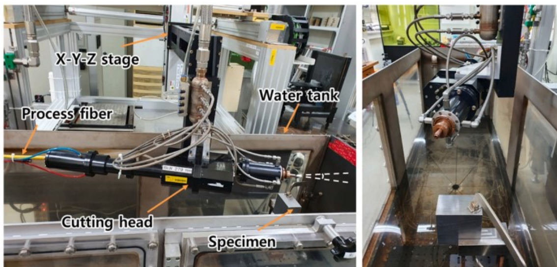
Slika 25. Prikaz podvodnog lasera za kutno rezanje
