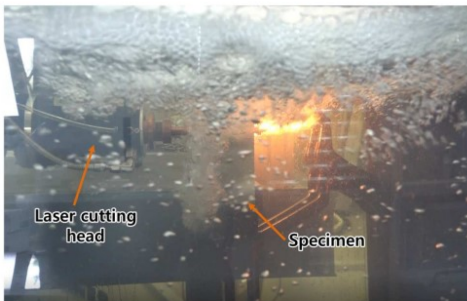
Slika 17. Prikaz procesa podvodnog rezanja laserom
