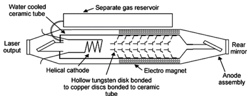
Slika 8. Prikaz sheme argonskog lasera
