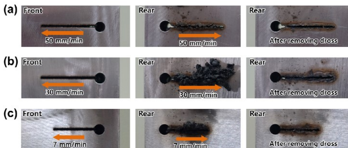
Slika 20. Prikaz uzoraka na kojima se primijenilo početno bušenje
