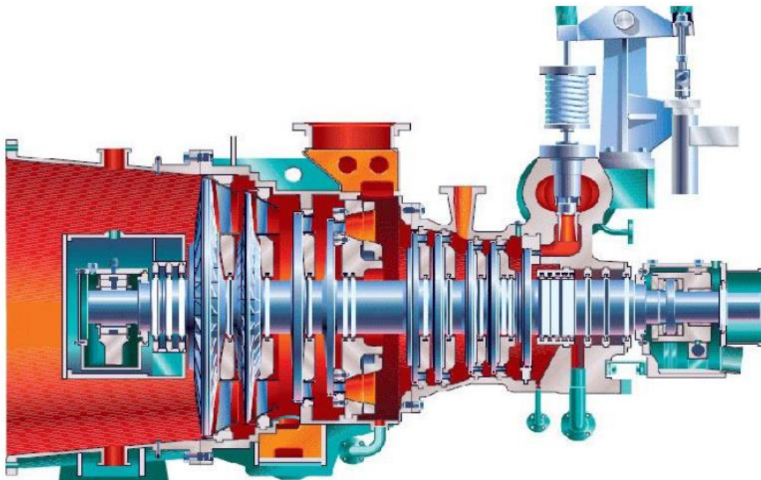
Slika 11. Parna turbina [16]
