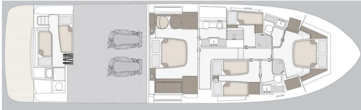
Slika 28: Tlocrt donje palube Azimuta 66
