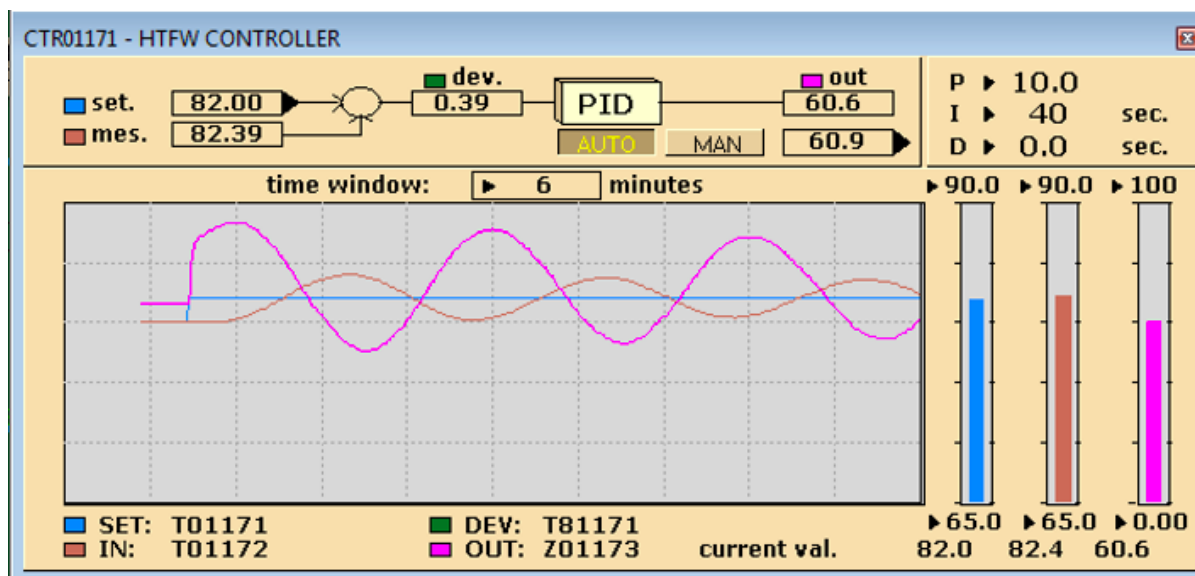
Slika 15. PI regulator [3]
