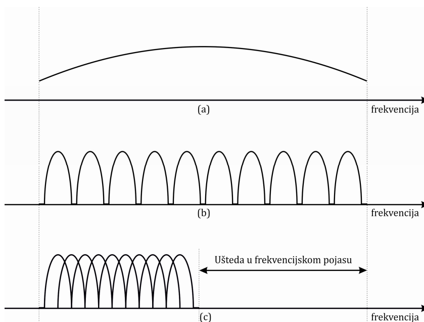
Slika 2: Usporedba sustava s jednim valom nosiocem (a), FDM modulacijom (b) i OFDM modulacijom (c)
