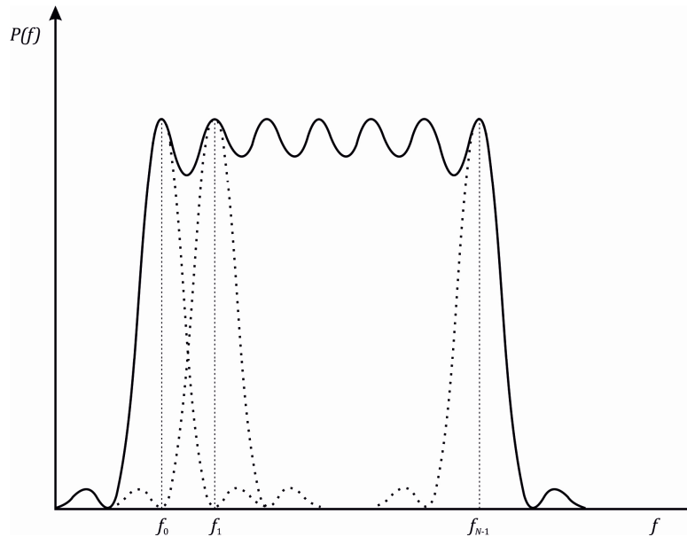
Slika 4: Spektralni dijagram snage OFDM signala
