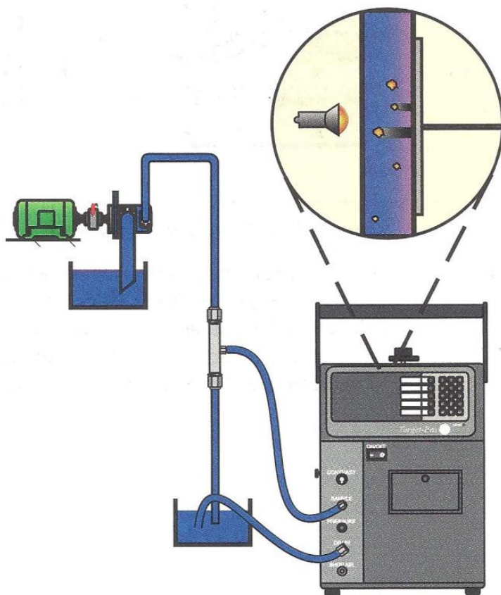
Slika 8 Automatski brojač čestica sa senzorom koji koristi bijelu svijetlost
