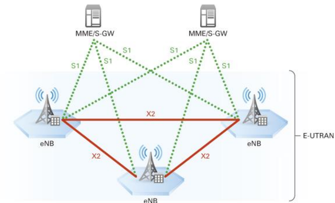
Slika 1. E-UTRAN Arhitektura
