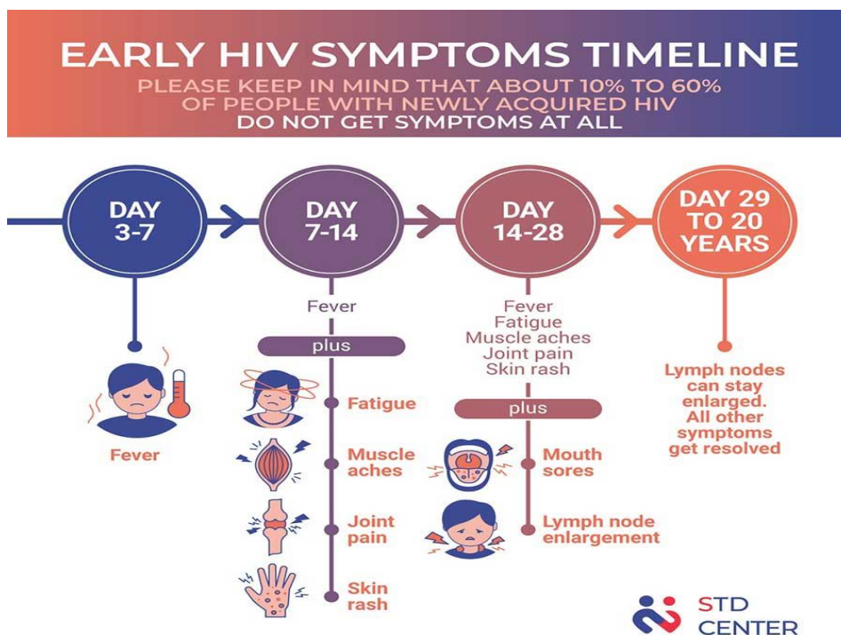
Slika 5. HIV simptomi
