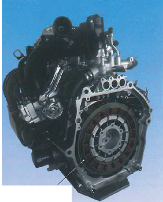
Slika 5.8. Ugradnja elektromotora između motora i mjenjača [50]
