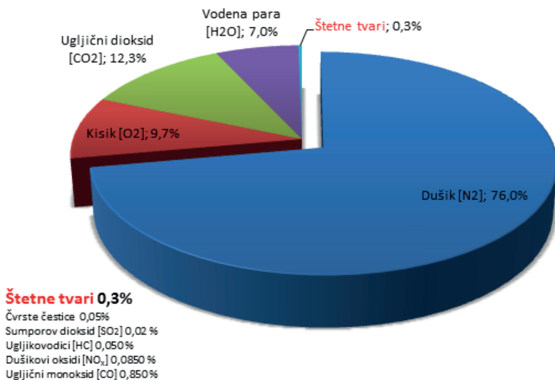
Slika 5.3. Sadržaj ispušnih plinova dizelskog motora [50]
