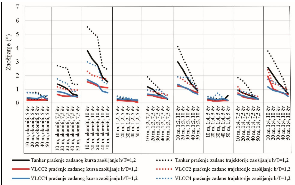
Grafikon 4: Odnos zaošijanja brodova punije forme kod postavke autopilota na praćenje zadanog kursa ( head ) i praćenja zadane trajektorije ( track ) za odnos h/T = 1,2
