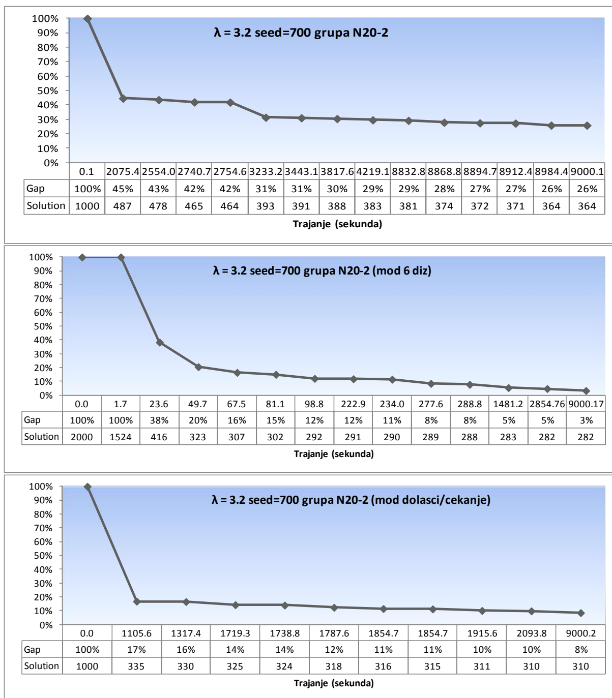
Slika 47: Graf procesa dobivanja optimalnog rješenja za slučaj N20-2 s tri varijacije
