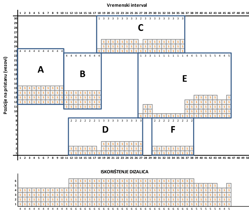
Slika 15: Rješenje integriranog BAP i QCAP problema
