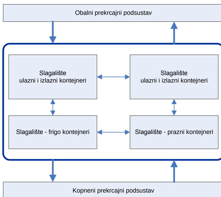
Slika 3: Zone kontejnerskog terminala i tijek procesa
