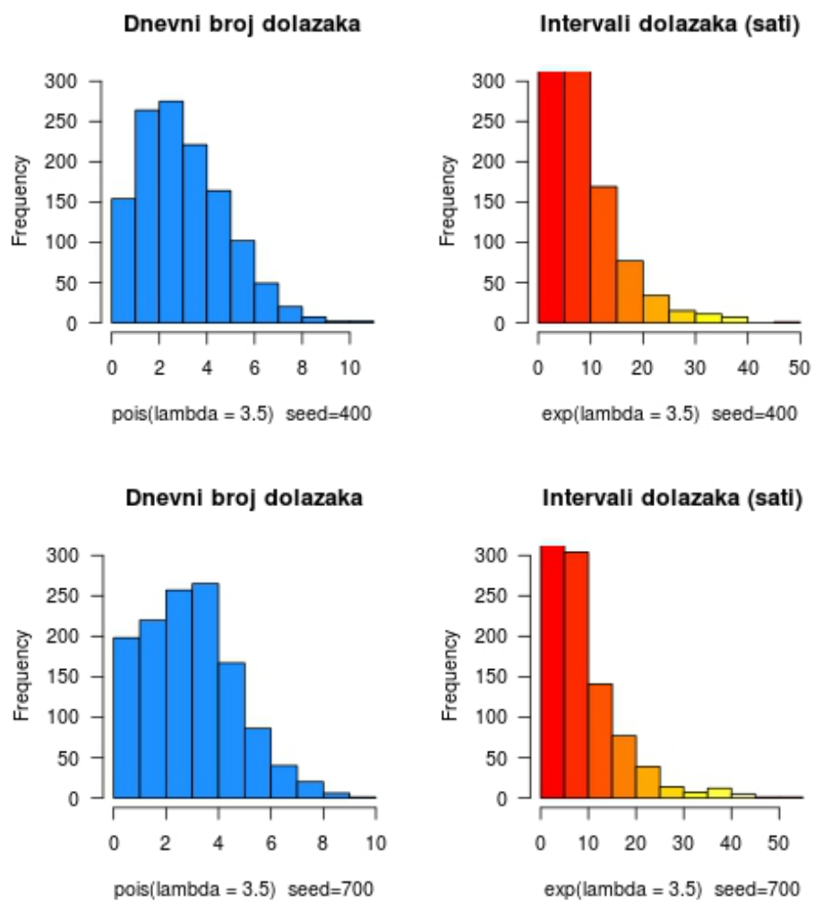
Slika 34: Frekvencija dolazaka brodova dobivena simulacijom za \lambda=3.5
