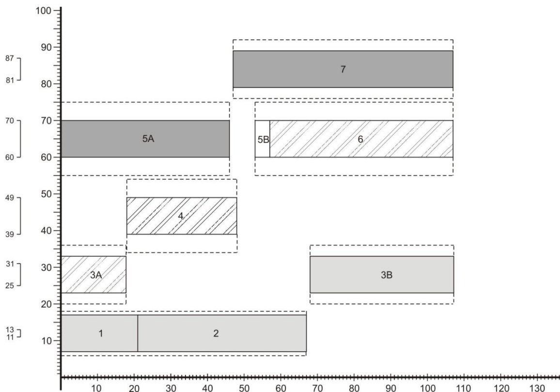
Slika 22: Rješenje QCSP problema s jednosmjernim kretanjem dizalica uz dijeljenje zadataka
