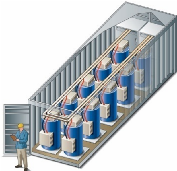
Slika 34. Modularno skladište energije na bazi zamašnjaka smješteno unutar standardnog brodskog 20-stopnog kontejnera [108]
