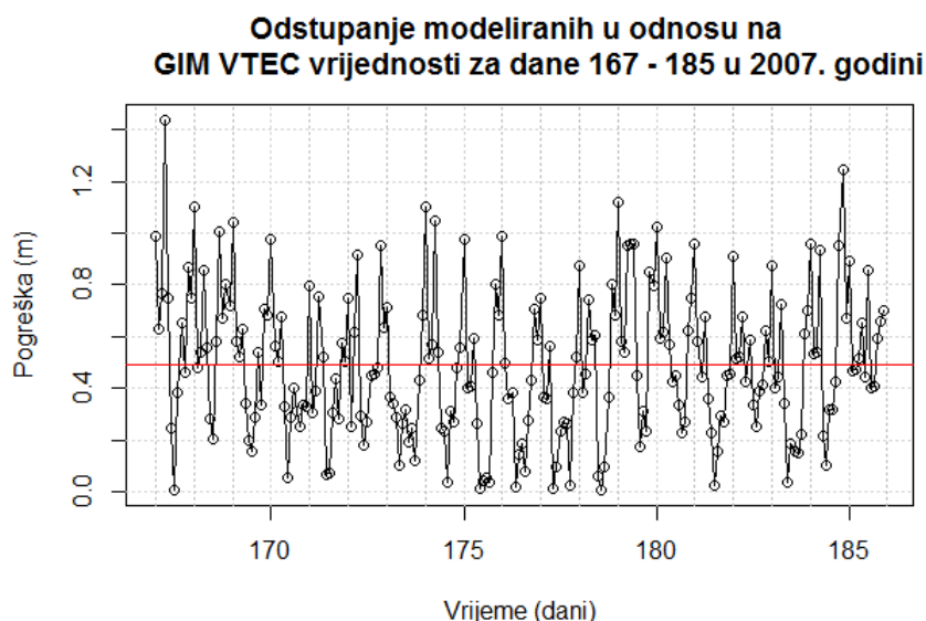
Slika 6.32: Prikaz odstupanja modeliranih u odnosu na GIM vrijednosti za dane 167 – 185 u 2007. godini uz naznačenu srednju vrijednosti odstupanja
