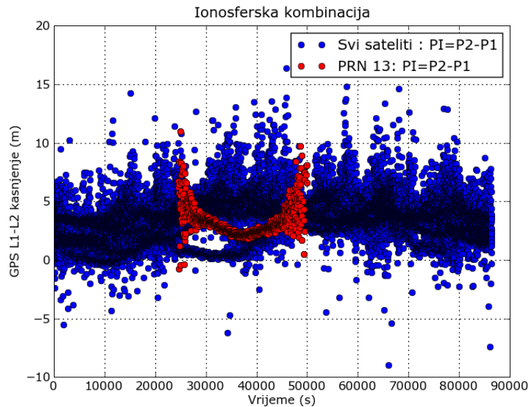
Slika 4.4: PI ionosferska kombinacija tijekom jednog dana kod prolazaka svih satelita, odnosno kod prolaska satelita PRN 13
