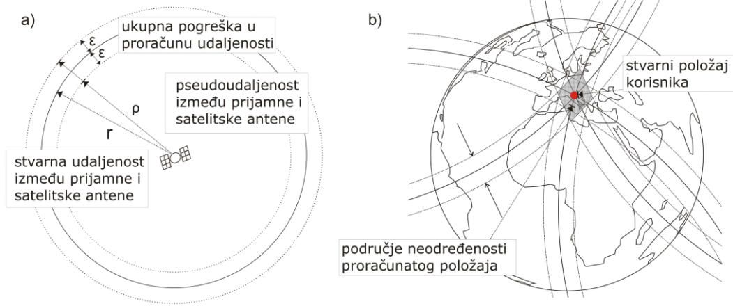
Slika 2.5: Prikaz stvarne udaljenosti i izmjerene pseudoudaljenosti između prijamne i satelitske antene (a) te područja neodređenosti proračunatog položaja (b)
