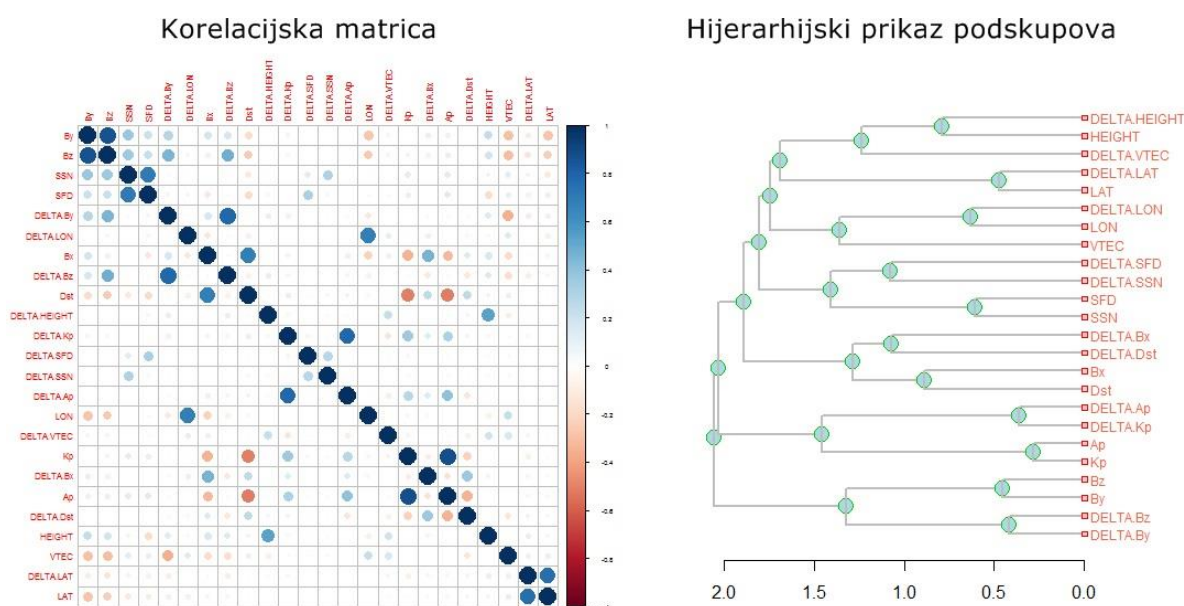
Slika 5.3: Korelacijska matrica pokazatelja svemirskog vremena (lijevo) i hijerarhijski prikaz (dendrogram) podskupova (desno)
