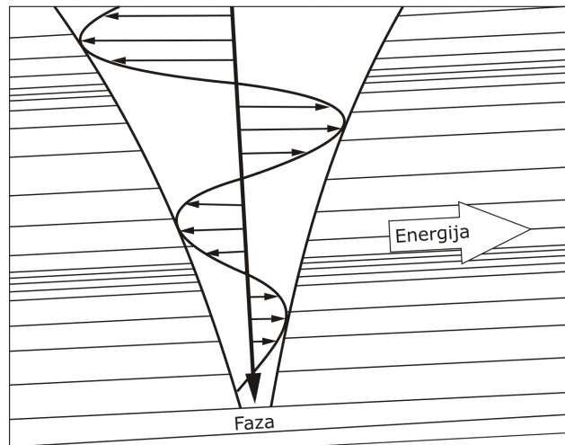
Slika 2.16: Shematski dijagram značajki širenja gravitacijskih valova Strelicama je prikazana promjena brzine širenja s visinom, dok blago nakošene linije prikazuju promjene u gustoći. Prikazan je smjer kretanja valne grupe (energija) te fazne brzine gravitacijskih valova
