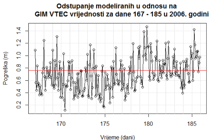
Slika 6.29: Prikaz odstupanja modeliranih u odnosu na GIM vrijednosti za dane 167 – 185 u 2006. godini uz naznačenu srednju vrijednost odstupanja
