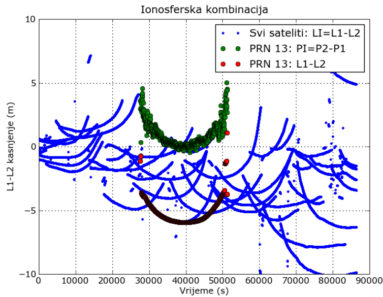
Slika 3.6: Značajke GPS kodnih i faznih dvofrekvencijskih mjerenja
