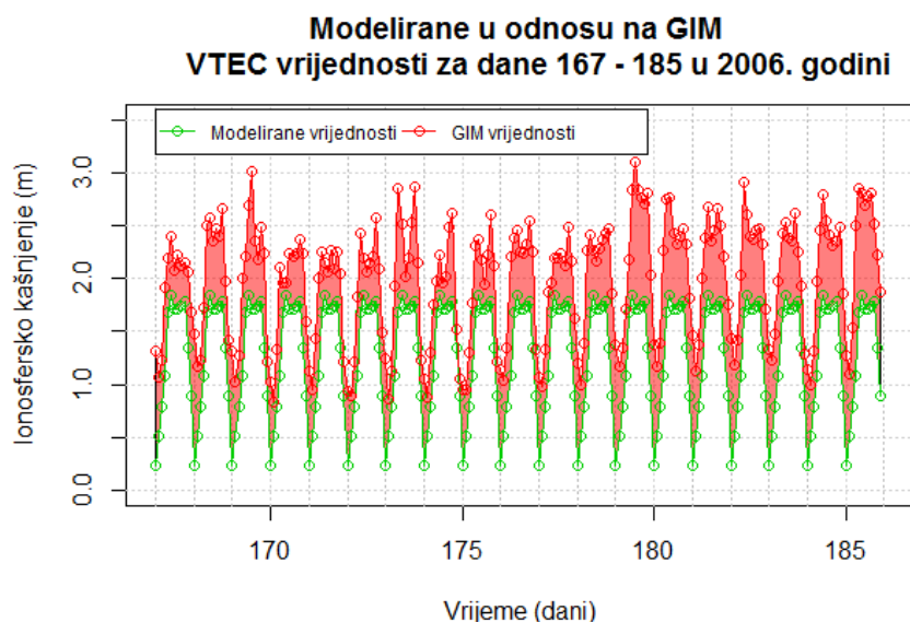
Slika 6.28: Prikaz modeliranih i GIM vrijednosti ionosferskog kašnjenja za dane 167 – 185 u 2006. godini
