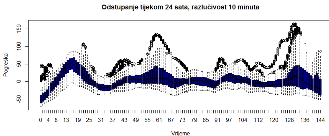
Slika 7.5: Regionalno relativno odstupanje (u %) predloženog modela od stvarnih vrijednosti ionosferskog kašnjenja tijekom 24 sata, prikazano s vremenskom razlučivošću skupova podataka od 10 minuta
