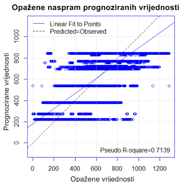
Slika 5.8 Opažene naspram prognoziranih vrijednosti slobodnog sadržaja elektrona izražene u (TECU/100) – primijenjeni prognostički model
