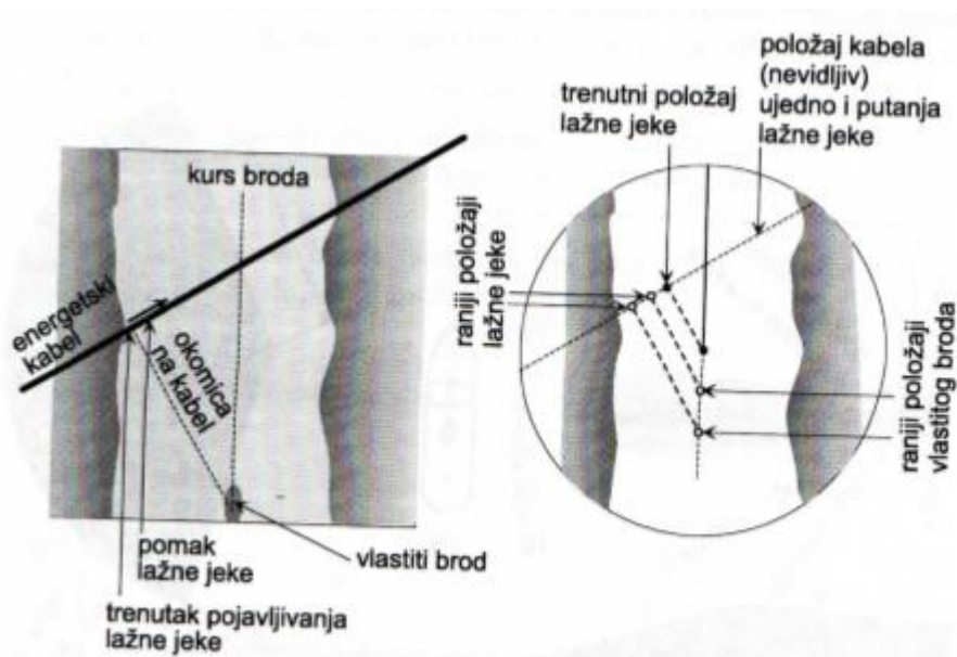
Slika 13. Lažne jeke nastale međudjelovanjem radarskog signala i energetskog kabela
