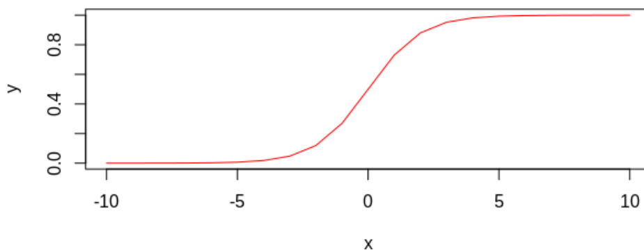
Slika 26. Sigmoidna funkcija
