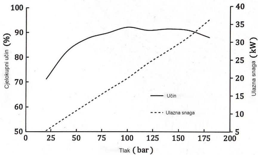
Dijagram 5.3 - Cjelokupni učin zupčaste pumpe pri brzini od 1500 0/min
