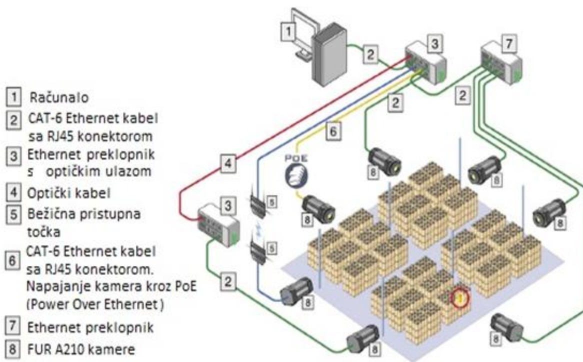
Slika 52: Tipična konfiguracija sustava vatrodjave pomoću termovizijskih kamera
