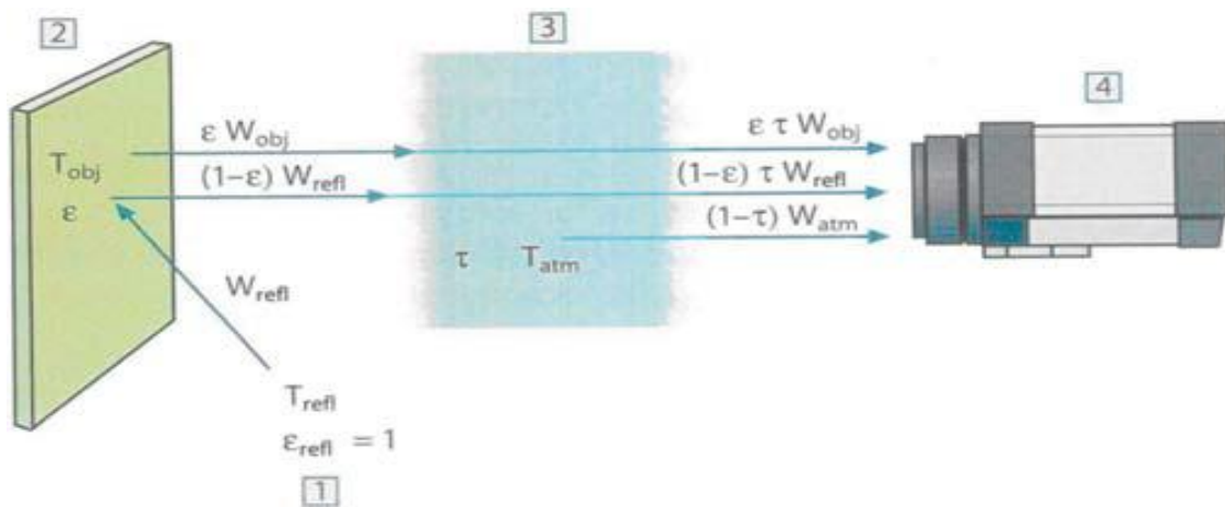
Slika 48: Shematski prikaz općeg termografskog mjerenja 1-okolinu; 2-objekt; 3-atmosfera; 4-kamera
