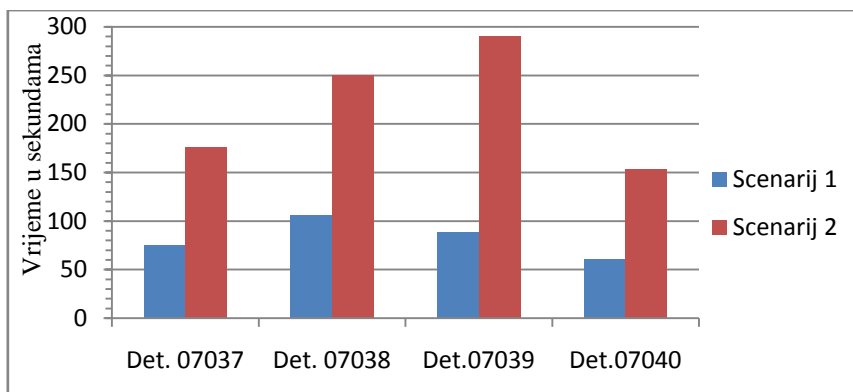
Grafikon 10 : Usporedba vremena alarma detekcije dima s (scenarij 1) i bez uključene ventilacije strojarne (scenarij 2)
