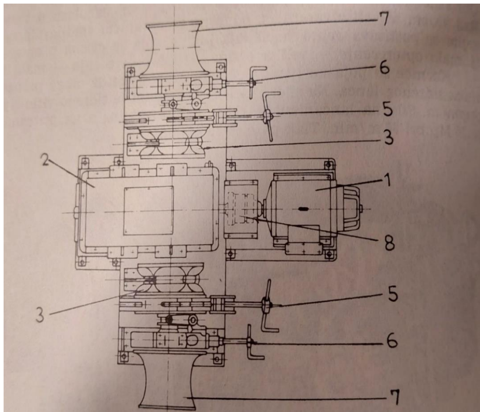
Slika 9-Prikaz sidrenog vitla na električni pogon
