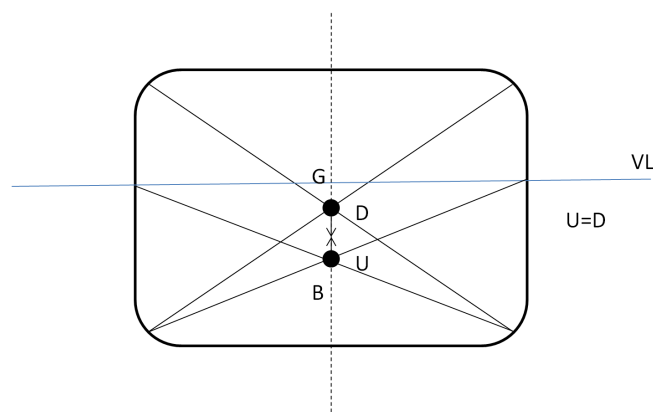
Slika 11. Prikaz drugog uvjeta plovnosti
