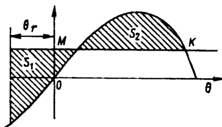
Slika 23. Prikaz momenata prevrtanja koristeći krivulju statičke stabilnosti
