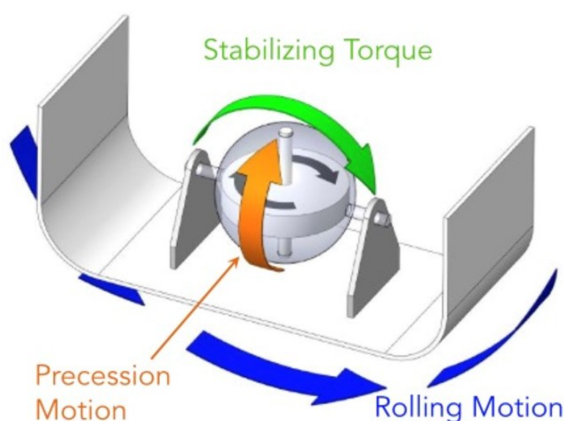
Slika 28. Prikaz sustava žiro stabilizatora
