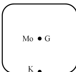
Slika 19. Prikaz indiferentnog broda
