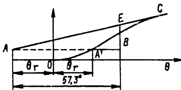
Slika 22. Prikaz momenta prevrtanja koristeći krivulju dinamičke stabilnosti
