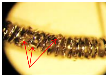
Slika 2. Spiralno vlakno sa istopljenim staklenim fragmentima iz staklenog balona (levo) i bliži pogled na istopljene fragmente stakla (desno)
