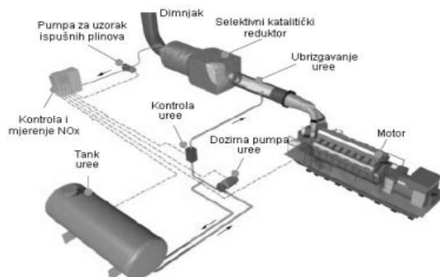
Slika 4: Šema selektivne katalitičke redukcije[9]
