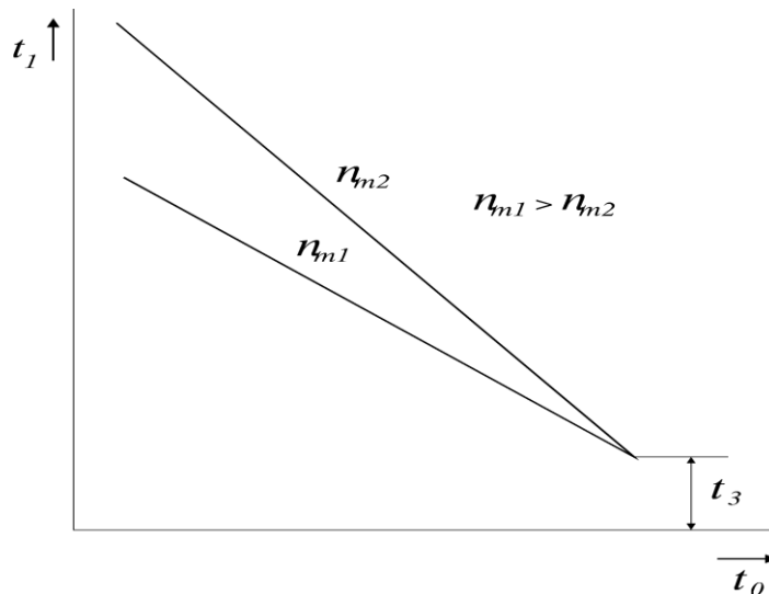
Slika 14. Temperaturska karakteristika startovanja motora
