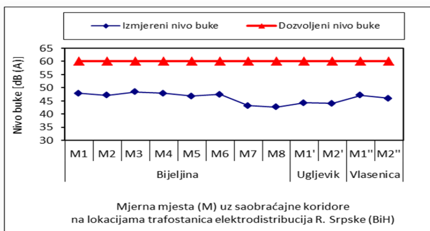
Slika 3. Rezultati mjerenja nivoa buke uz saobraćajne koridore na lokacijama trafostanica
