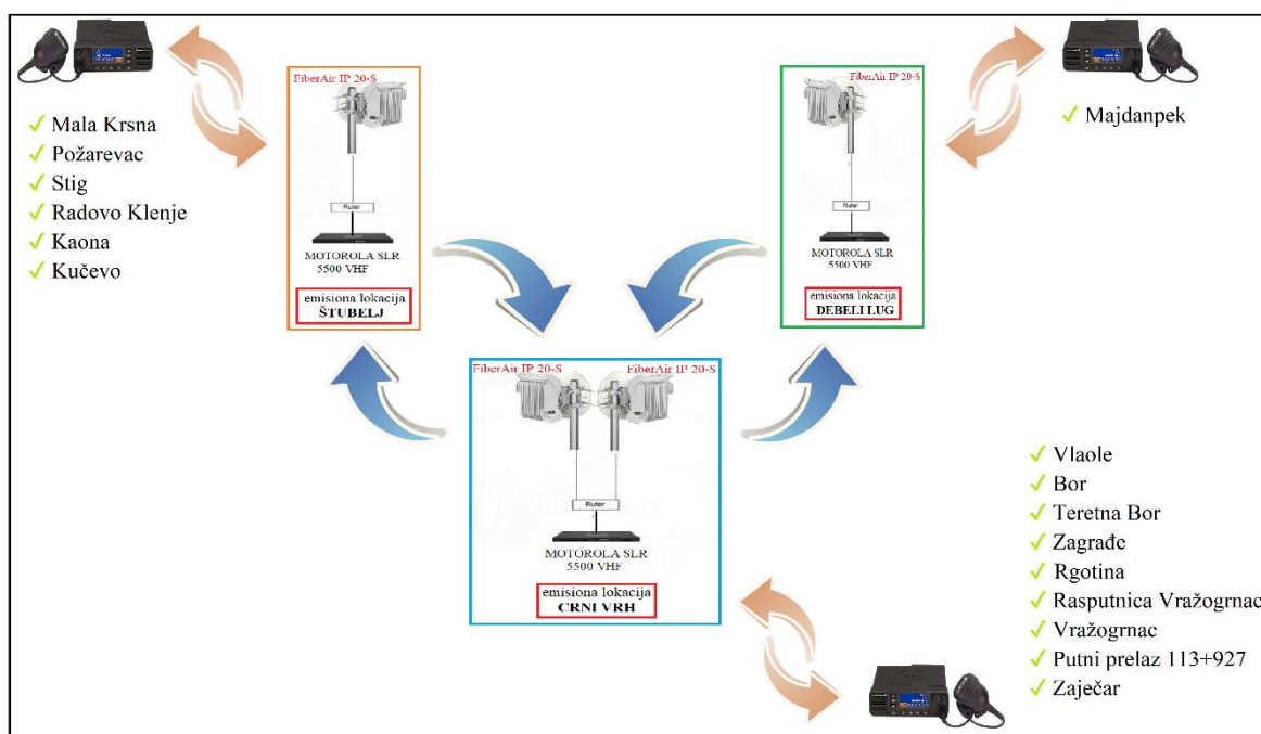
Slika 5. Blok šema predložene integrisane radio mreže na pruzama Mala Krsna - Požarevac - Bor - Vražogrnac i Crveni Krst - Zaječar - Prahovo Pristanište između Požarevca i Zaječara
