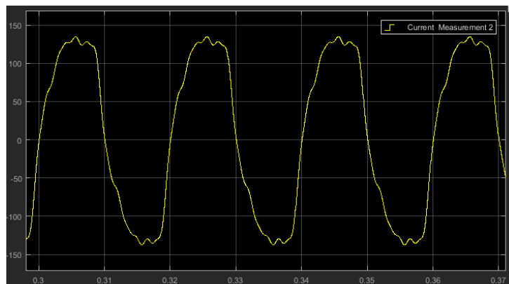
Slika 3. Vremenski dijagram struje faze L2
